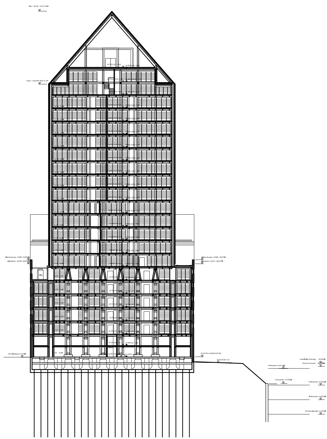
Schnitt A-A Speicher
