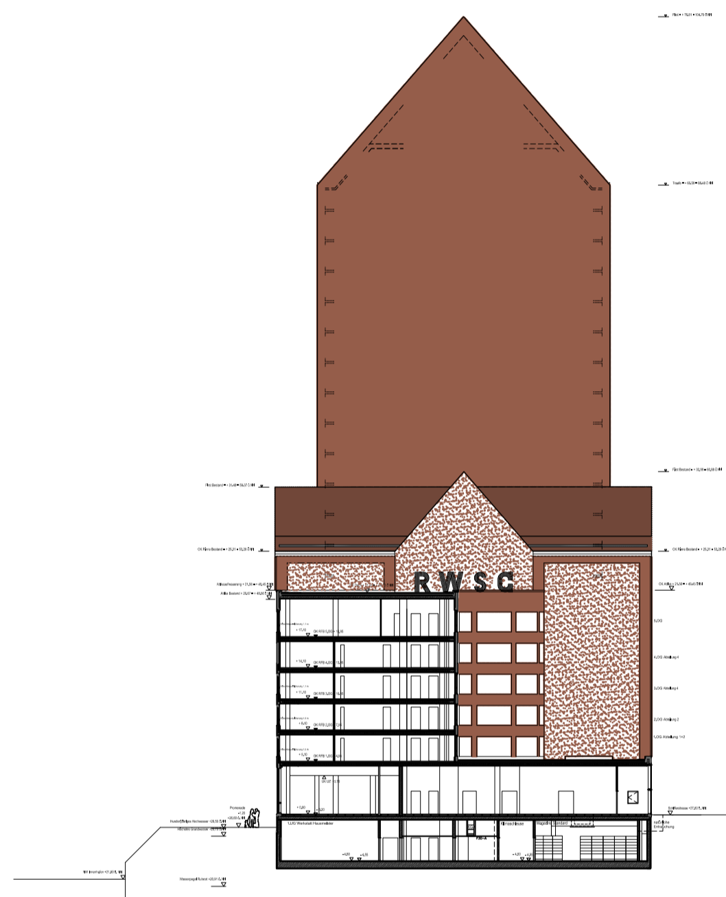
Schnitt B-B Welle
