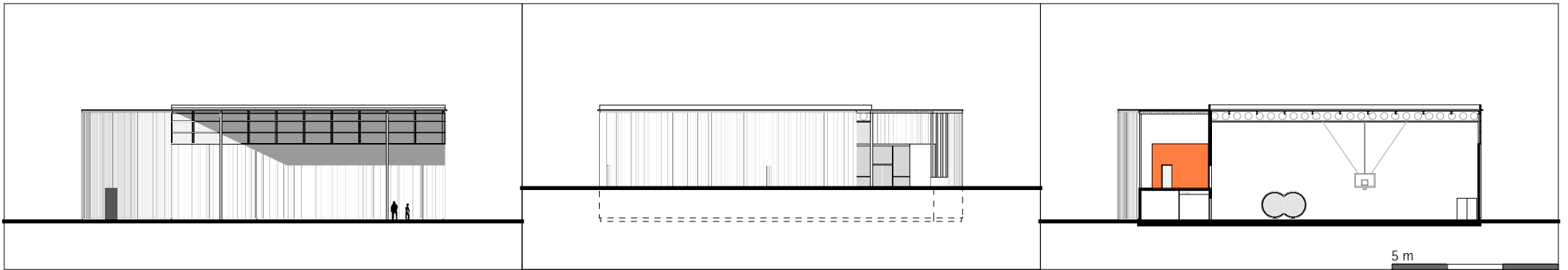
ELEVATION EST
