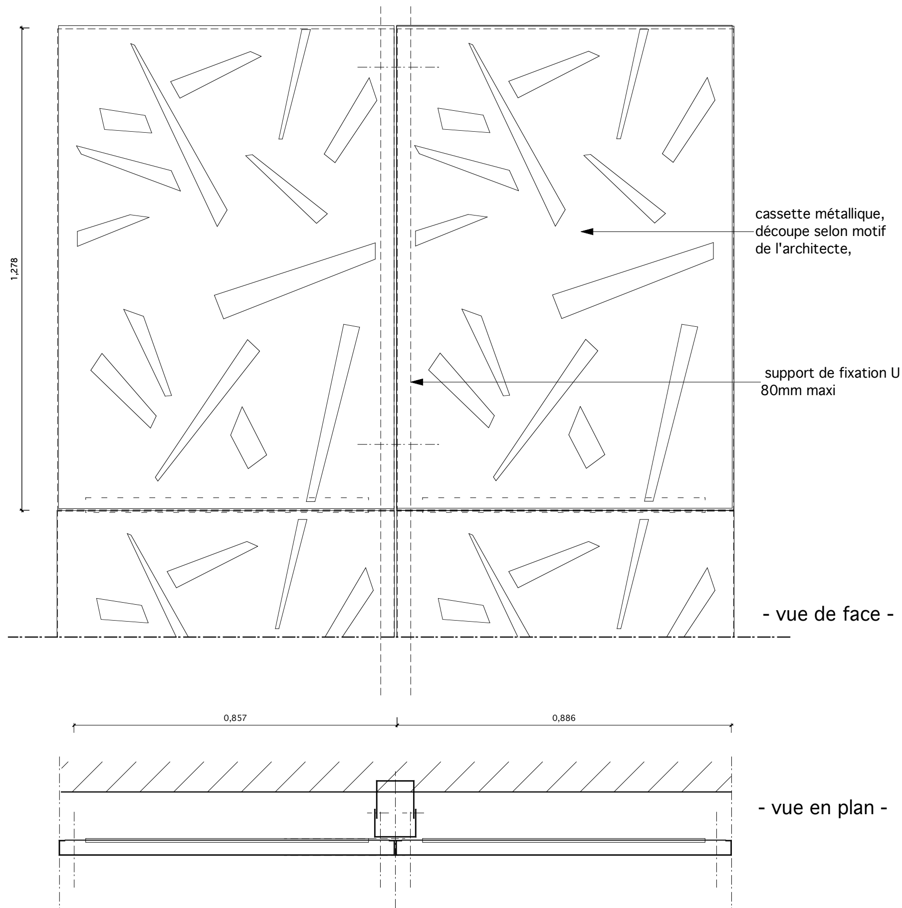
Principes de fixation des cassettes métalliques sur la structure du hall d'accueil - 1/10e
