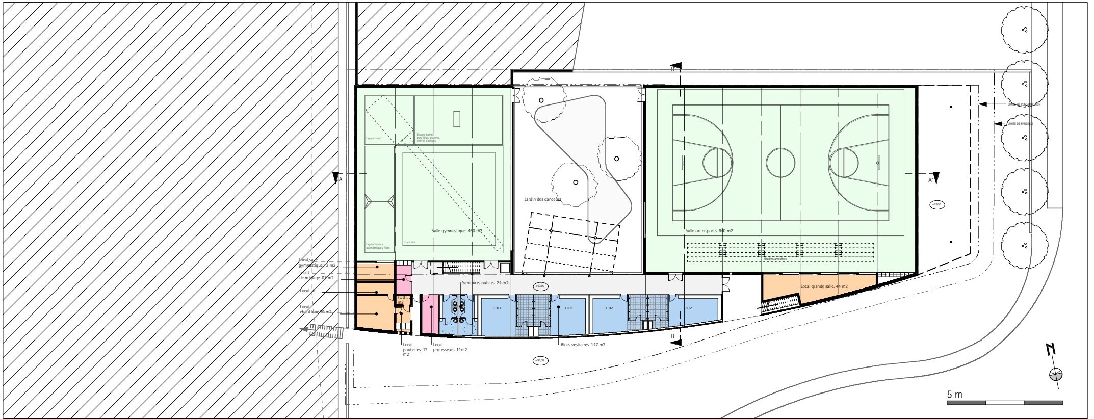
PLAN REZ DE CHAUSSEE
