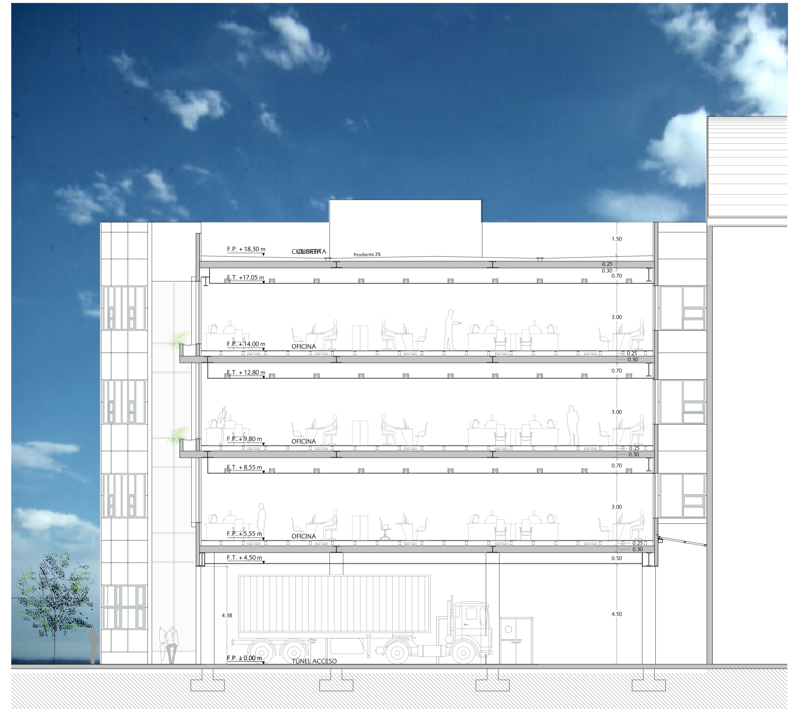
SECCION 4-4'
