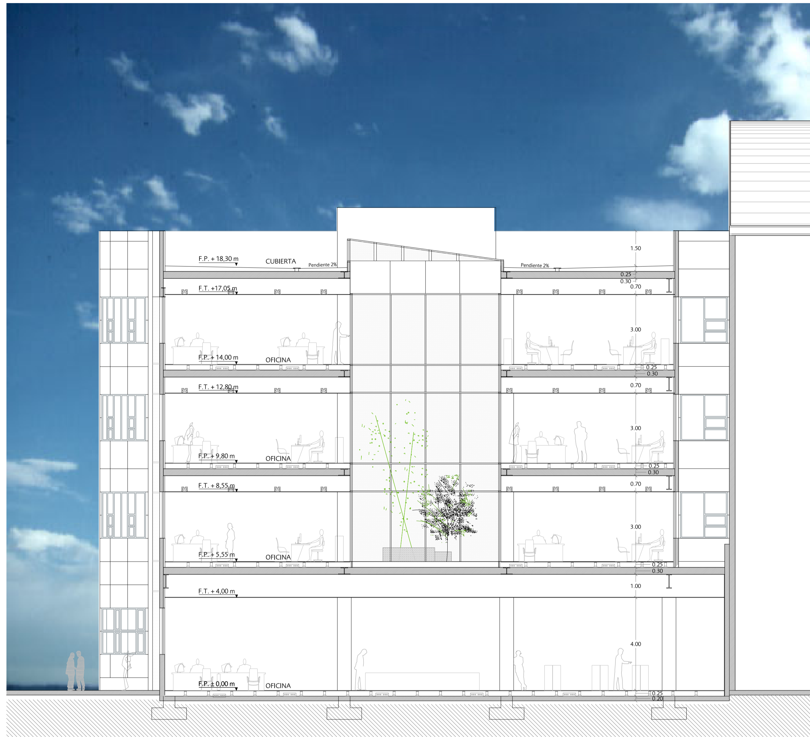
SECCION 3-3'
