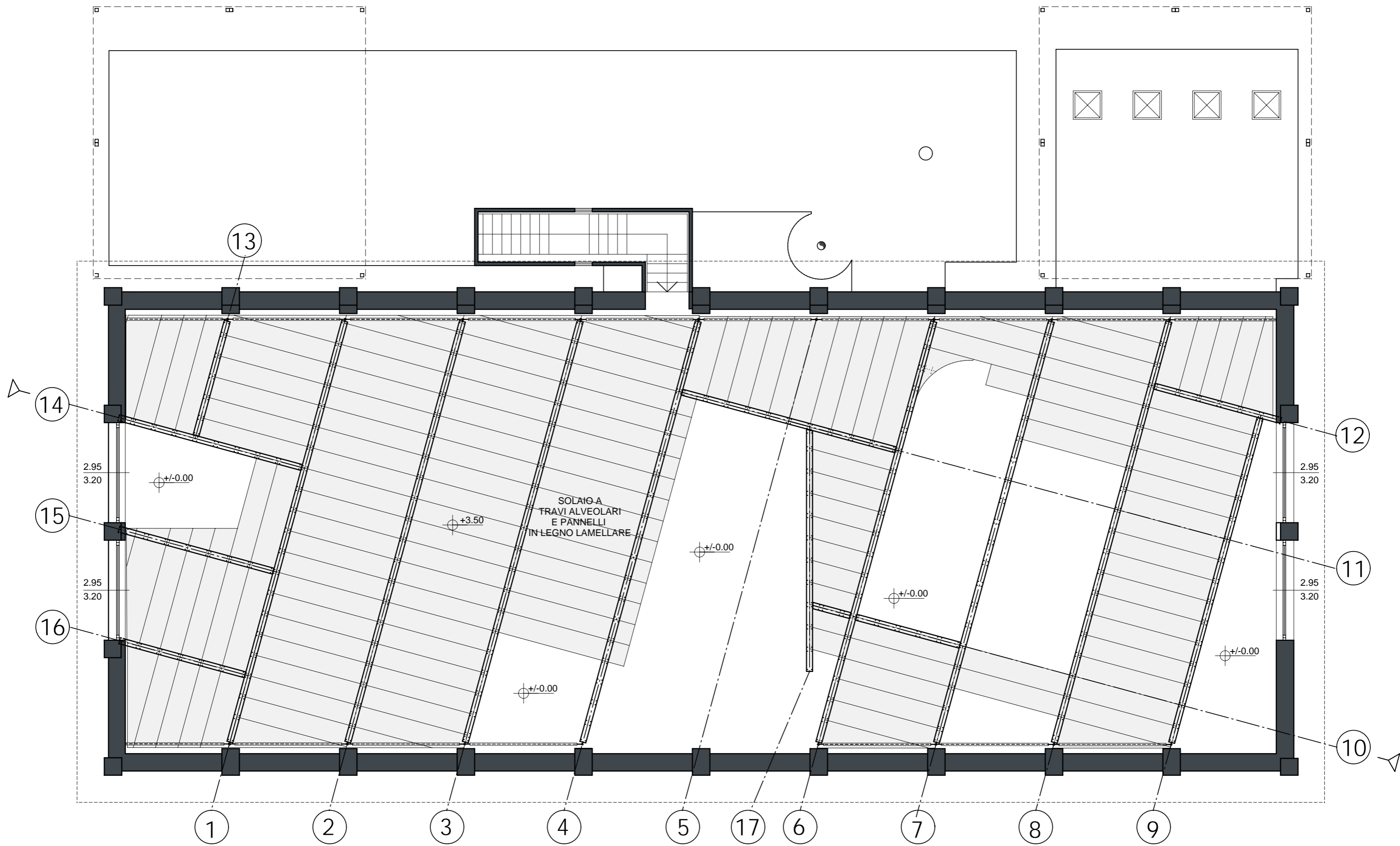
stato in progetto nuovo soppalco interno: solaio a travi alveolari e pannelli in legno lamellare
