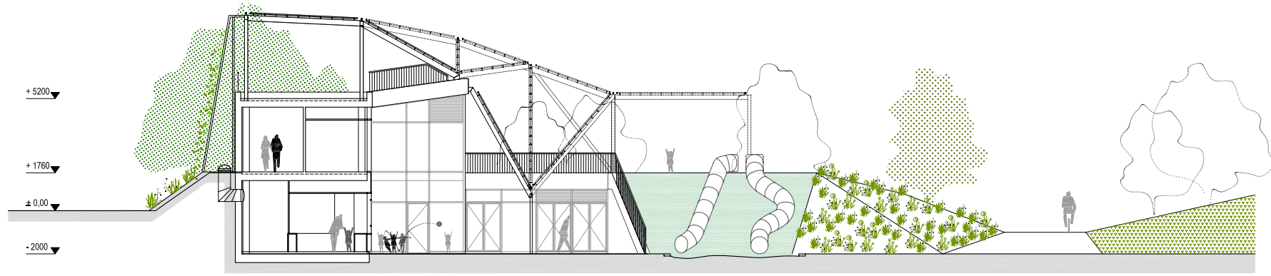
SECCIÓN B-B'
