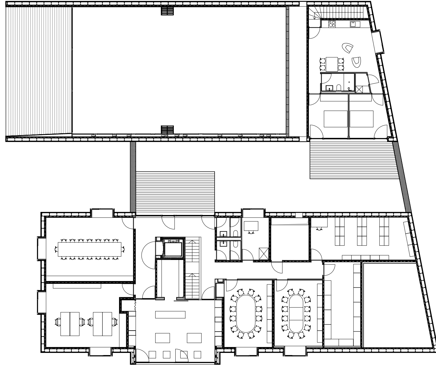
niveau +1 1:200
