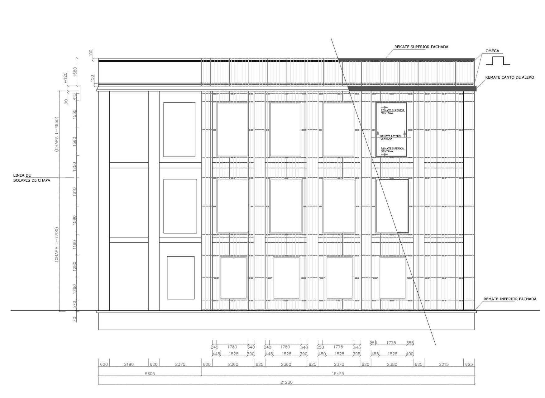
FACHADA OESTE
