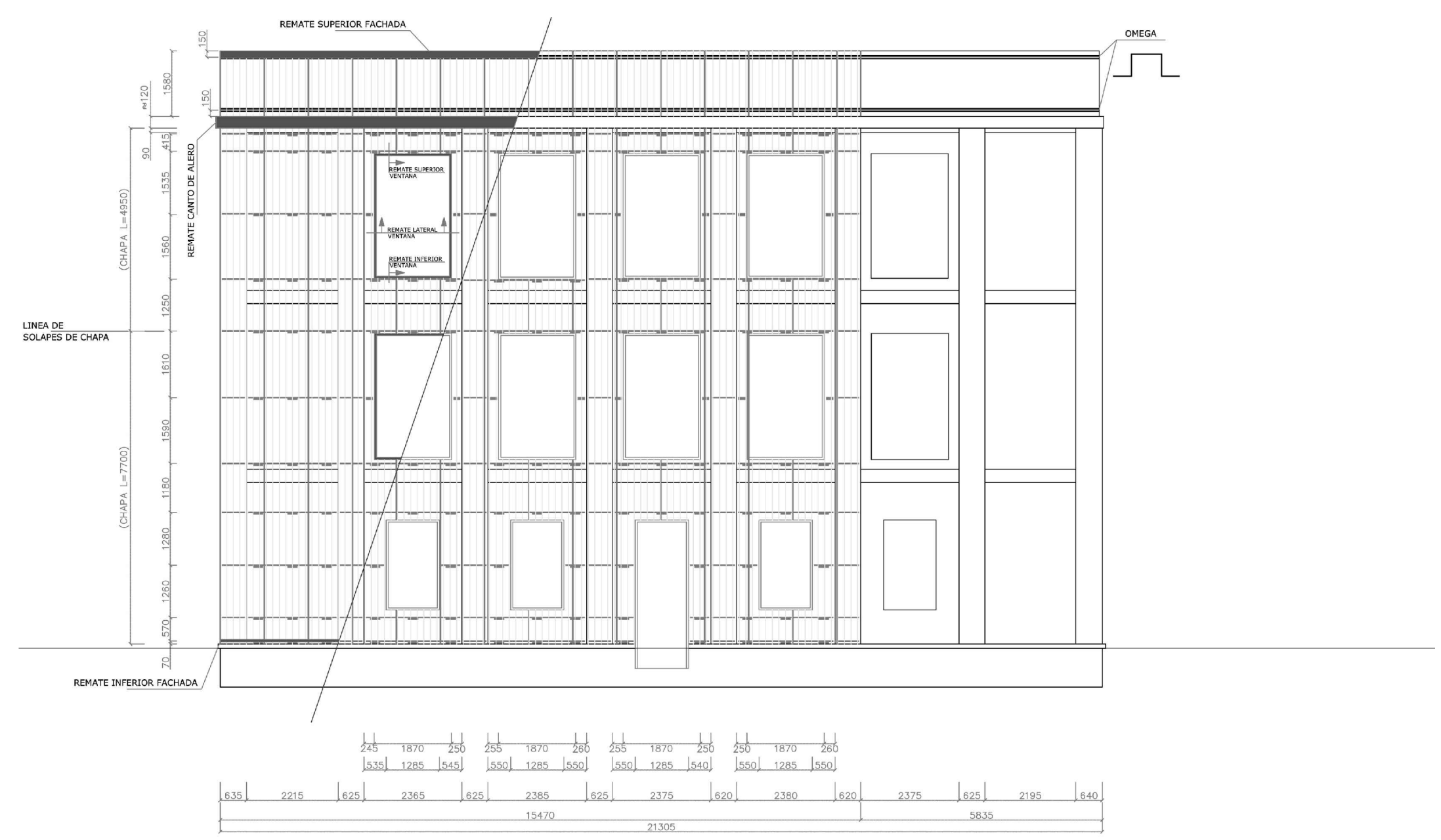
FACHADA ESTE
