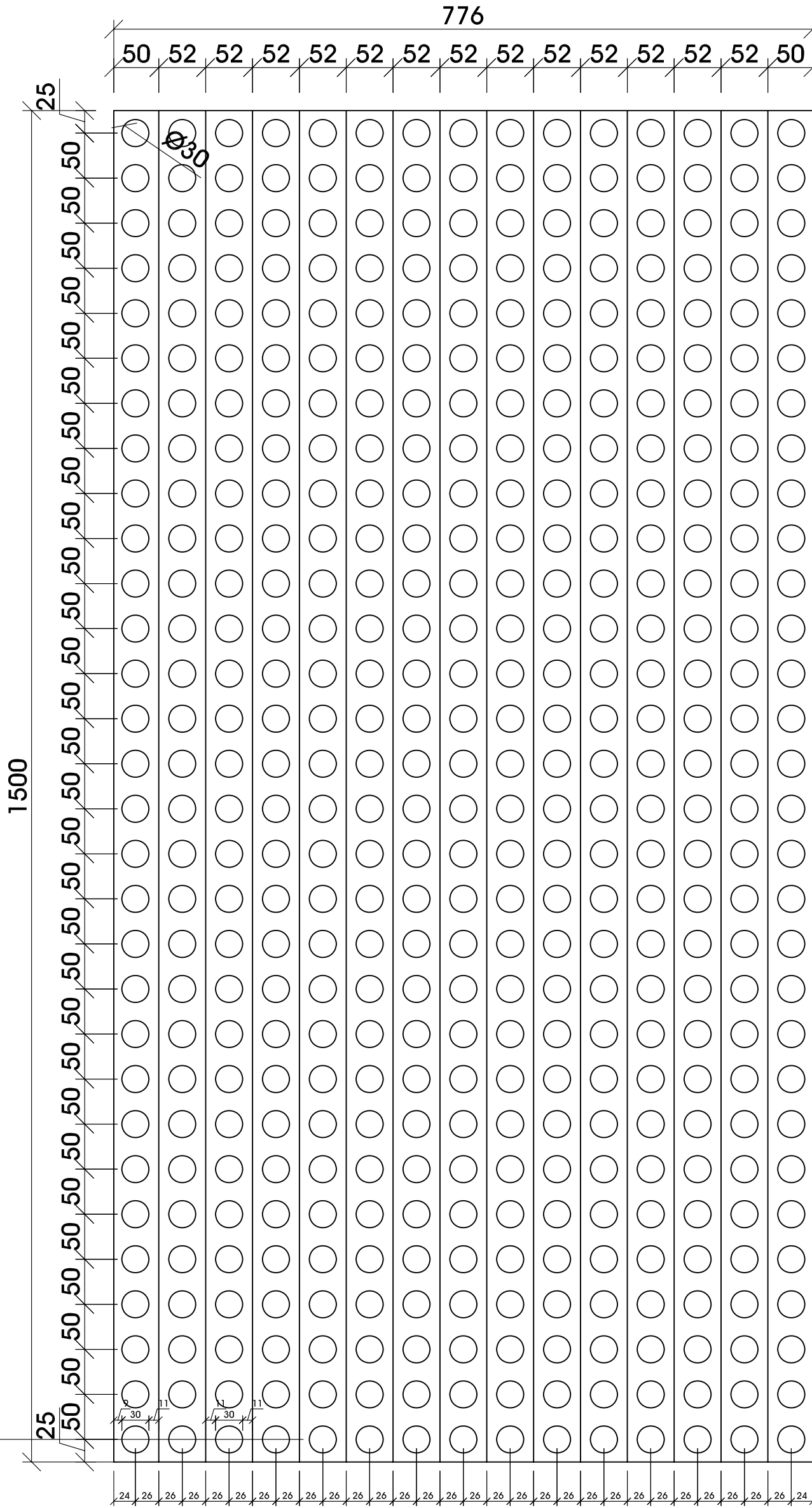
Aanzicht
